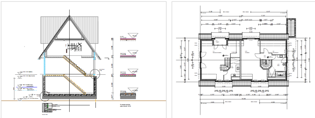
Skizzen und Grundrisse des Objektes (Bildnachweis: Architekturbüro Dipl.-Ing. M. Wolter)
